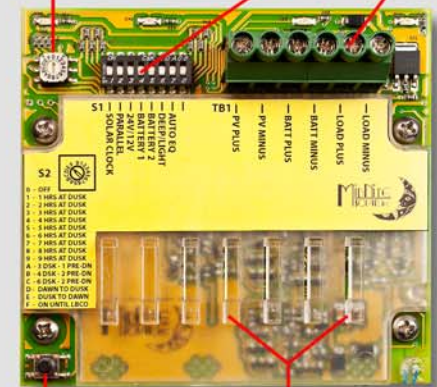
Charge / bouton de test Câble Serre-câbles
